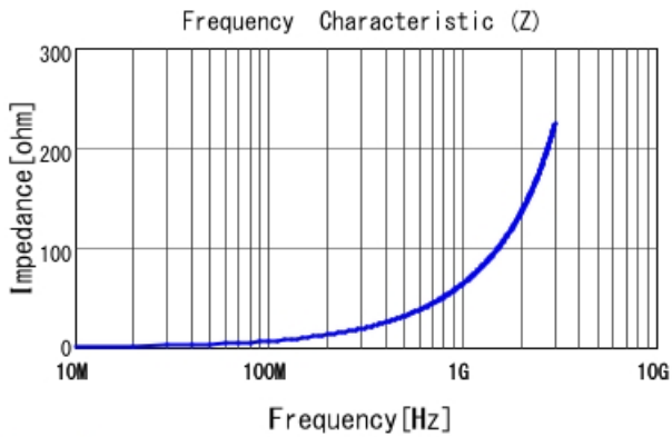
LQW18AN10NJ10 |Z|
