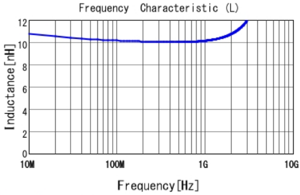
LQW18AN10NJ10 L
