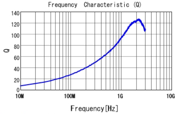
LQW18AN10NJ10 Q
