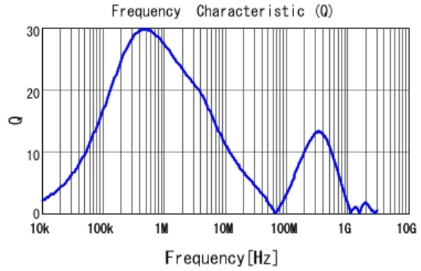
1229AS-H-4R7M Q
