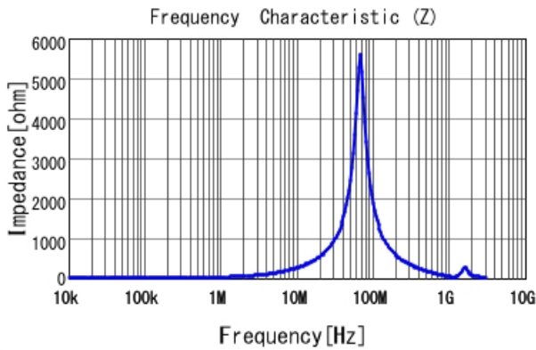
1229AS-H-4R7M |Z|
