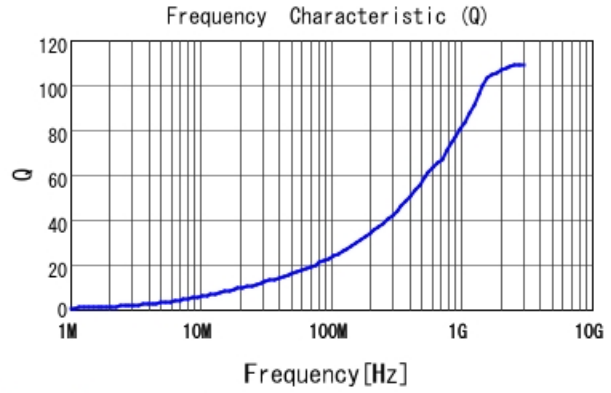
LQW15AN4N6G80 Q
