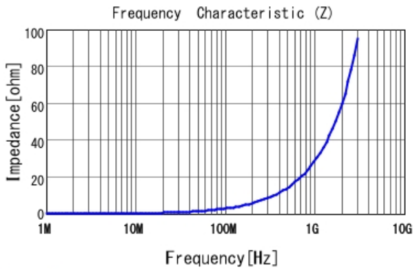
LQW15AN4N6G80 |Z|
