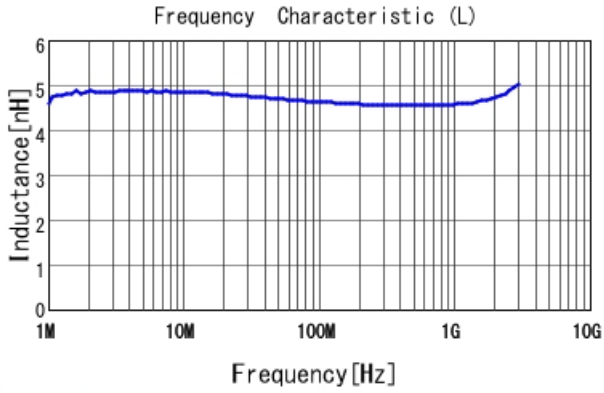
LQW15AN4N6G80 L
