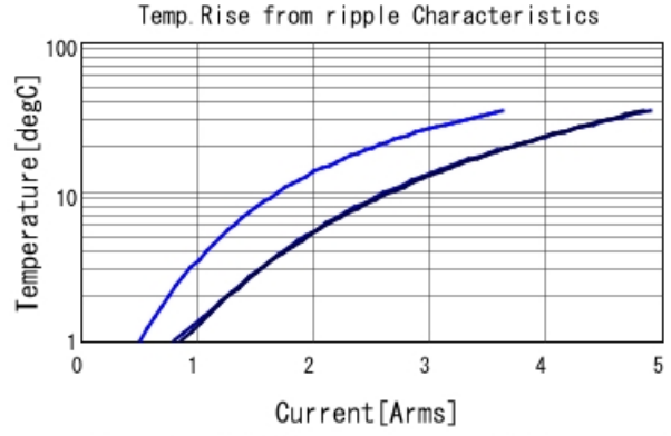
GRM319B31A106KE18 Temp. rise — 100kHz — 500
