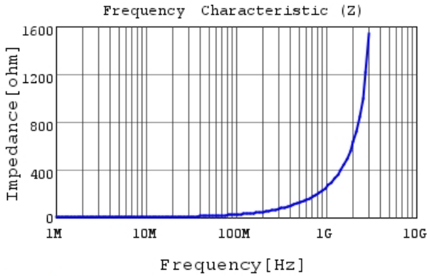
LQW15AN39NJ8Z |Z|
