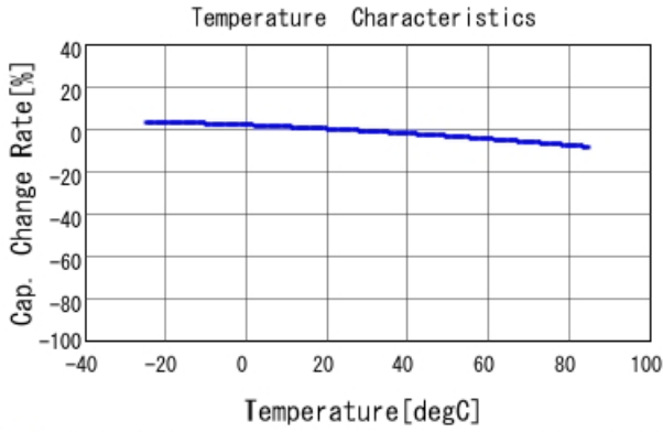
■ GRM033B10J103KA01 C-Temp. capchange, DCO. 0V, AC1. 0Vrm
