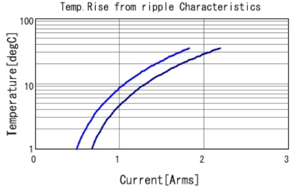
GRM152D70G224KE15 Temp. rise — 500kHz — 1MHz
