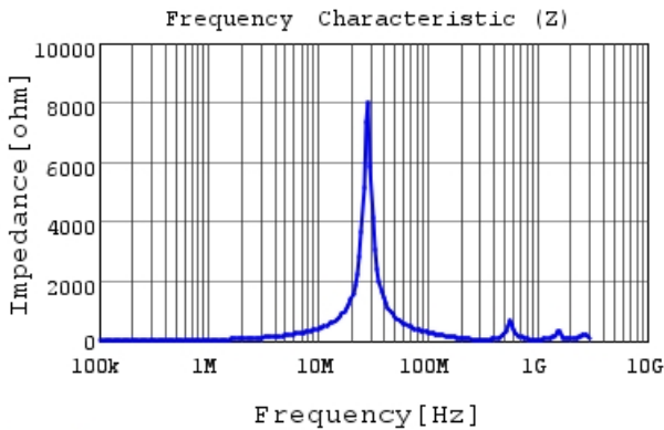
■ MDH7045C-6R8NB |Z|
