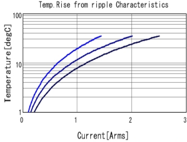
GRM188R71E474KA12 Temp. rise ■ 200kHz ■ 500kHz ■ 1MHz
