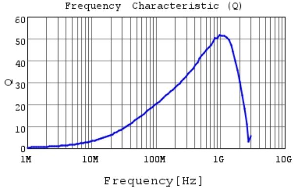
LQW15AN68NJ8Z Q
