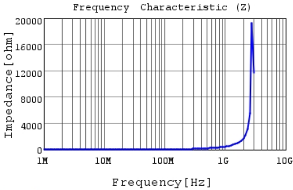
LQW15AN68NJ8Z |Z|
