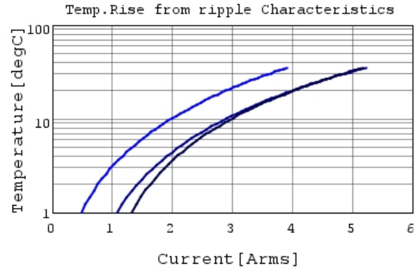
GRM188C80E106ME47 Temp.rise — 80kHz —
