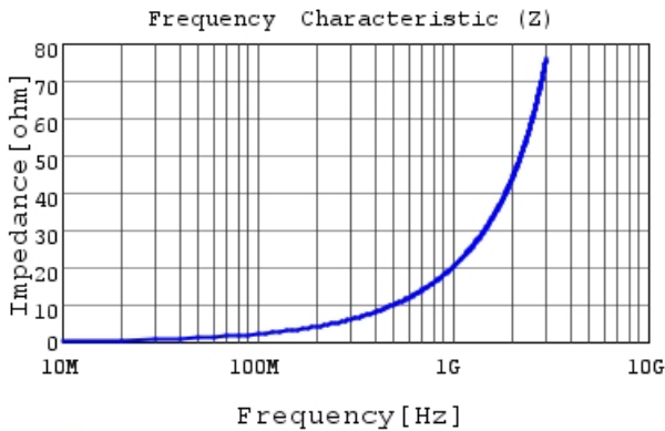
LQG15HZ3N3S02 |Z|
