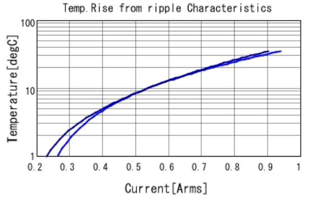
GQM2195C2E1R8BB12 Temp. rise — 2GHz — 3GHz
