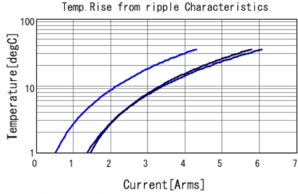
GRT21BC81A106KE01 Temp. rise — 80kHz — 400kHz
