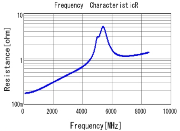
■ GRM0332C1H160JA01 R DCOV, 20degC
