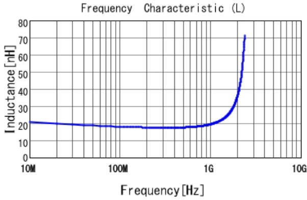
LQG15HN18NG02 L
