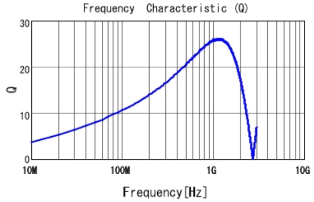
LQG15HN18NG02 Q
