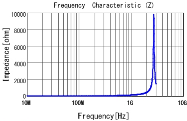
LQG15HN18NG02 |Z|
