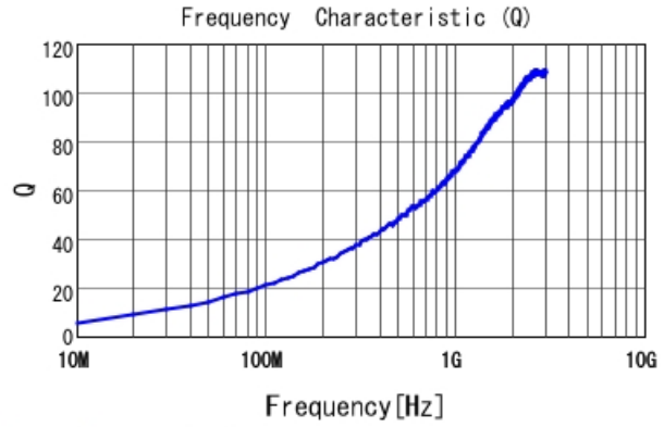
LQW15AN4N7D1Z Q
