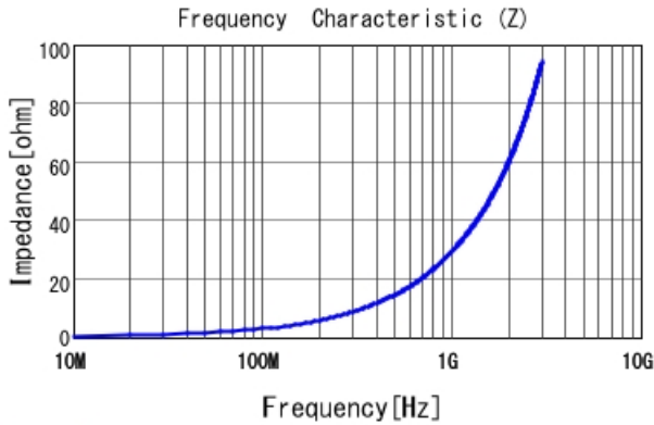
LQW15AN4N7D1Z |Z|
