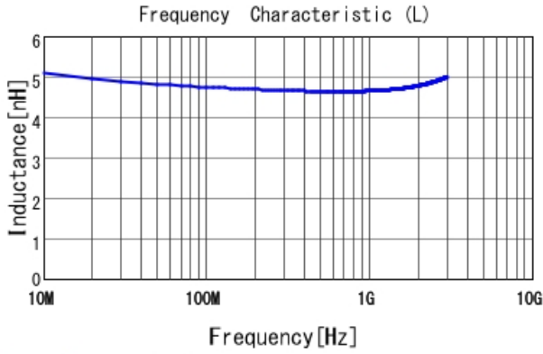
LQW15AN4N7D1Z L
