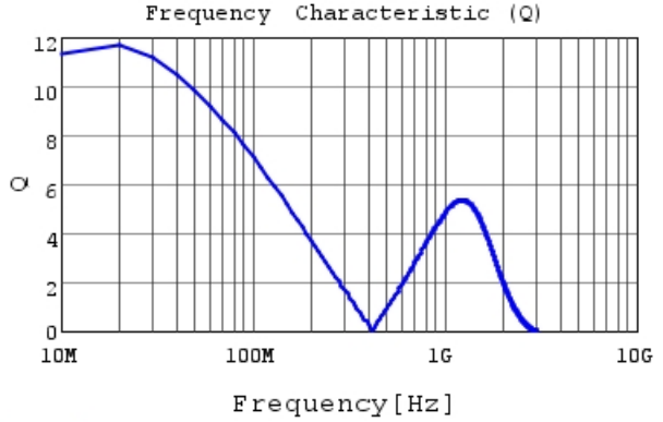
LQW15CNR56J1Z Q
