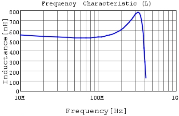
LQW15CNR56J1Z L
