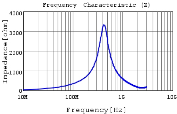
LQW15CNR56J1Z |Z|
