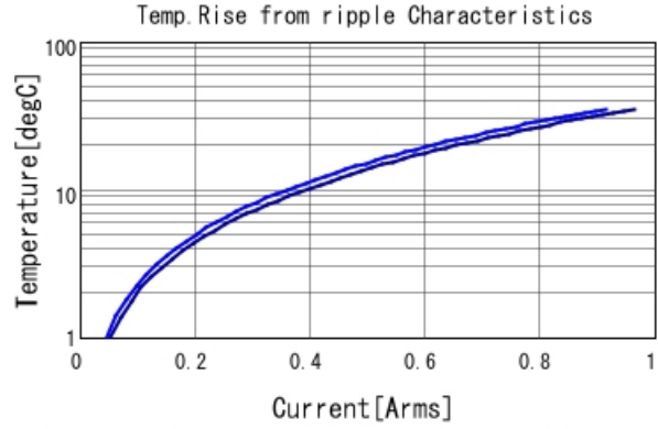
GRM033R61C104ME18 Temp. rise ■ 800kHz ■ 1MHz
