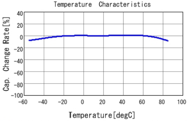
■ GRM033R61C104ME18 C-Temp. capchange, DCO. 0V, ACO. 5Vrm
