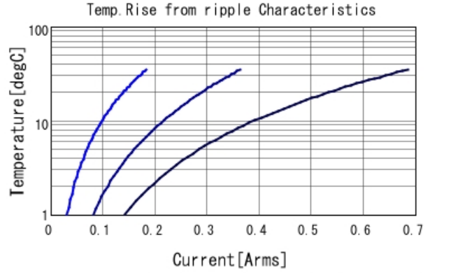
GCJ31CR72E333KXJ3 Temp. rise — 30kHz — 100kHz
