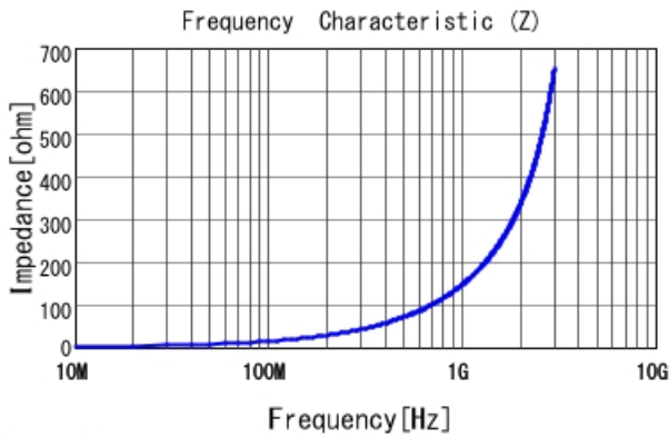
LQW15AN23NG00 |Z|
