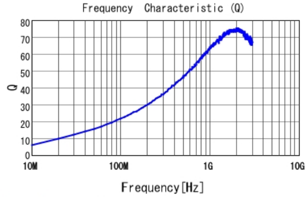
LQW15AN23NG00 Q
