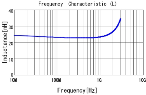
LQW15AN23NG00 L
