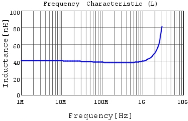
LQW15AN39NJ80 L
