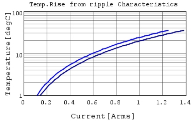
GRM033B30J224ME15 Temp.rise — 600kHz —
