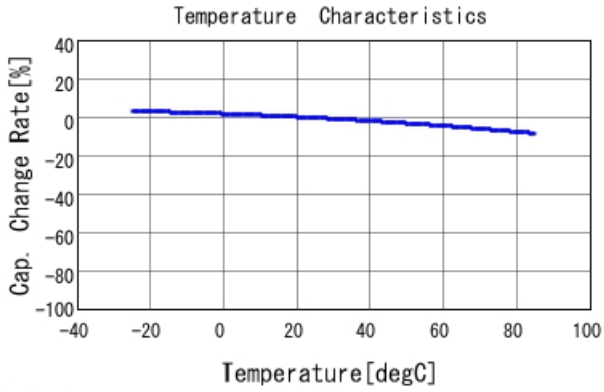
■ GRM033B31E103MA12 C-Temp. capchange, DCO. 0V, AC1. 0Vrm
