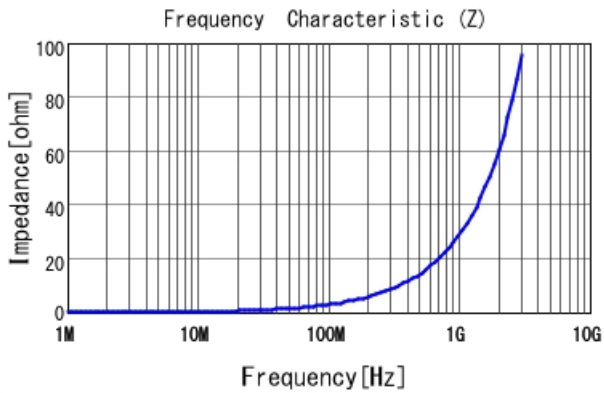
LQW15AN4N7C8Z |Z|
