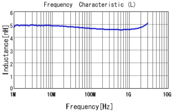
LQW15AN4N7C8Z L
