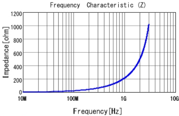
LQW15AN33NH0Z |Z|
