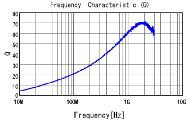
LQW15AN33NH0Z Q
