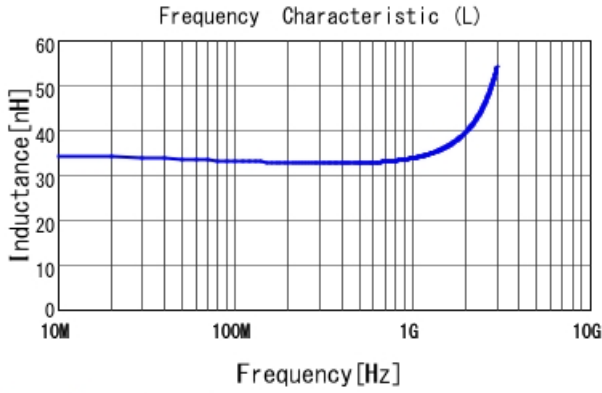
LQW15AN33NH0Z L
