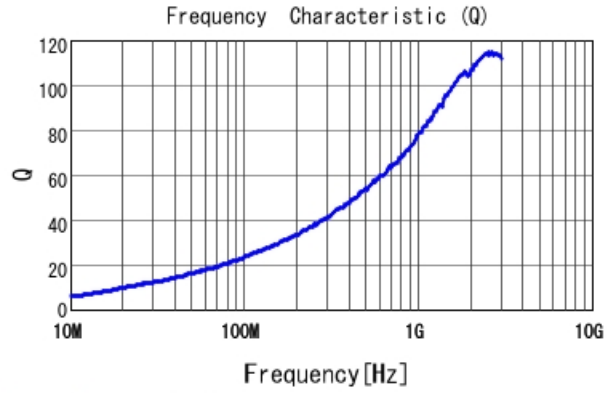
LQW18AN4N7C8Z Q
