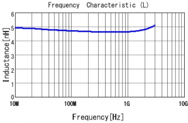
LQW18AN4N7C8Z L
