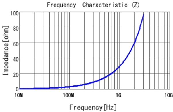
LQW18AN4N7C8Z |Z|
