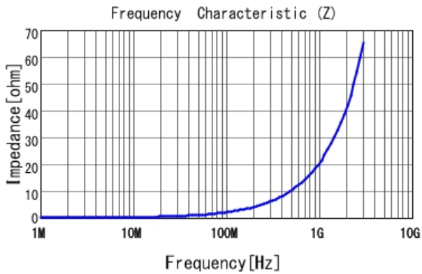
LQW15AN3N3D8Z |Z|
