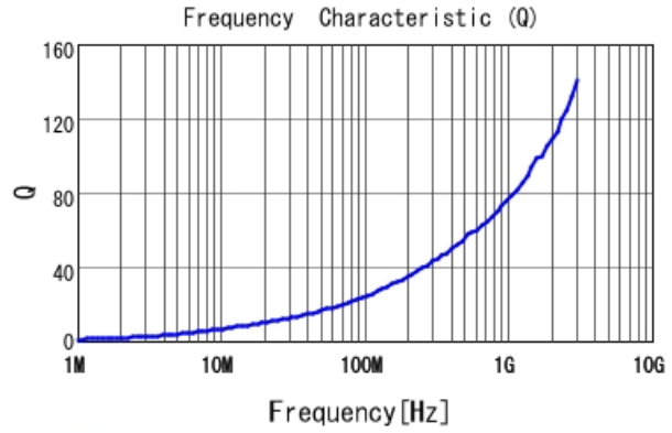
LQW15AN3N3D8Z Q
