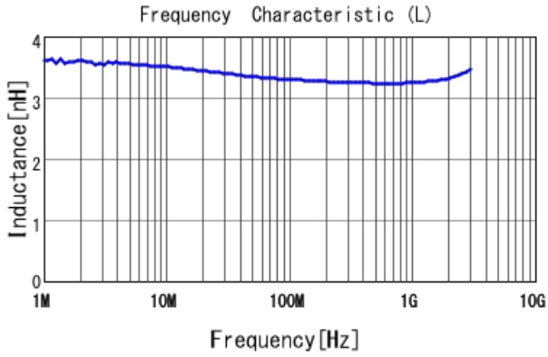
LQW15AN3N3D8Z L
