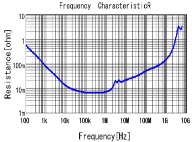
■ GRJ32ER71H106KE11 R DCOV, 25degC
