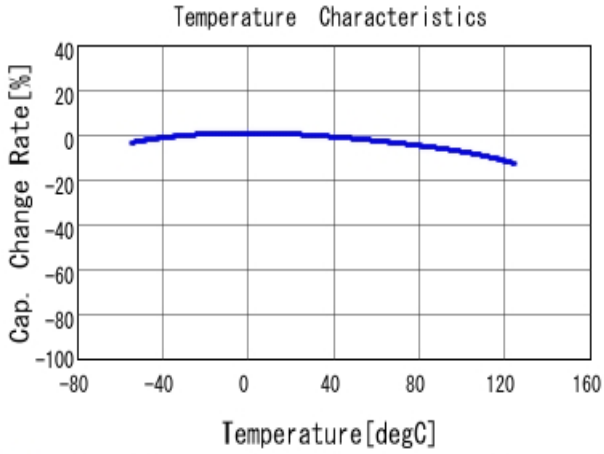
■ GRJ32ER71H106KE11 C-Temp. capchange, DCO. 0V, ACO. 1V rm
