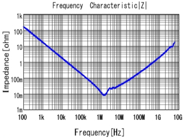
■ GRJ32ER71H106KE11 |Z| DCOV, 25degC
