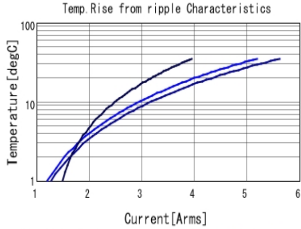
GRJ32ER71H106KE11 Temp. rise ■ 80kHz ■ 400kHz ■ 800kHz
