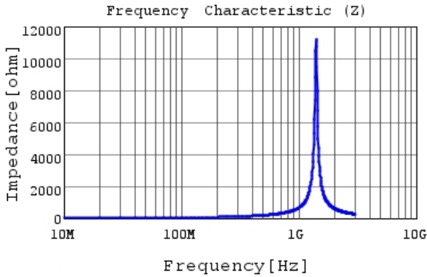
LQG15HN56NG02 |Z|
