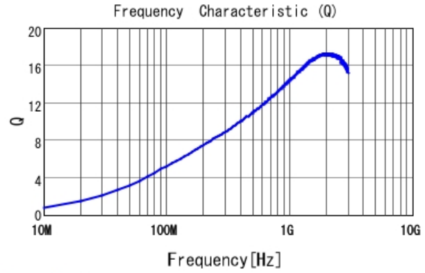
LQP02TQ18NH02 Q
