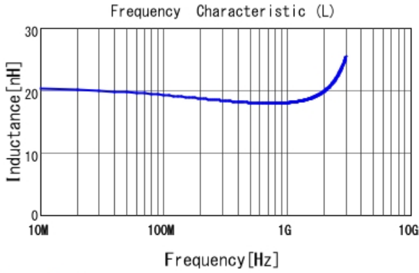
LQP02TQ18NH02 L
