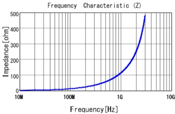
LQP02TQ18NH02 |Z|
