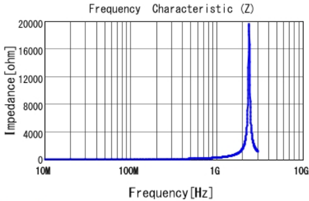
LQP03HQ39NH02 |Z|
