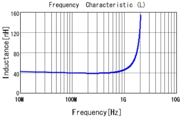
LQP03HQ39NH02 L
