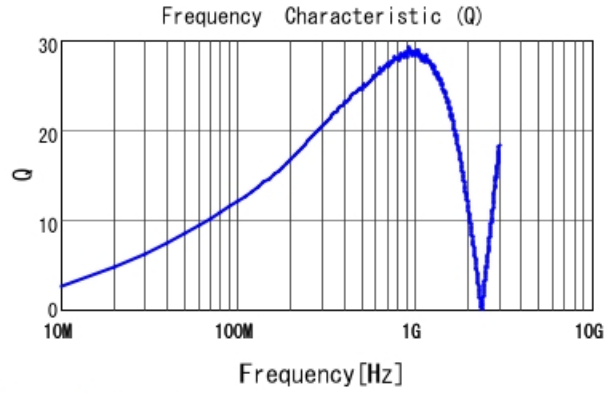
LQP03HQ39NH02 Q
