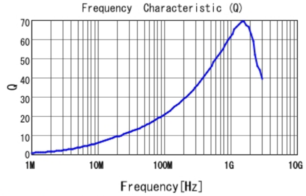
LQW15AN24NG80 Q
