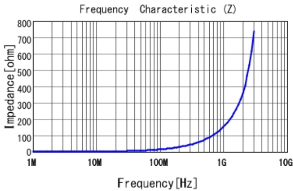
LQW15AN24NG80 |Z|
