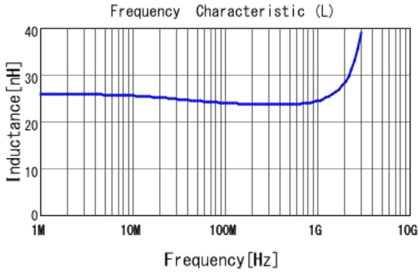
LQW15AN24NG80 L
