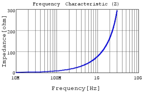
LQP02HQ12NH02 |Z|
