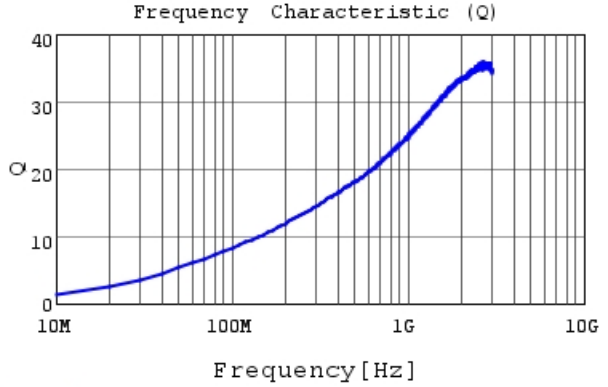
LQP02HQ12NH02 Q
