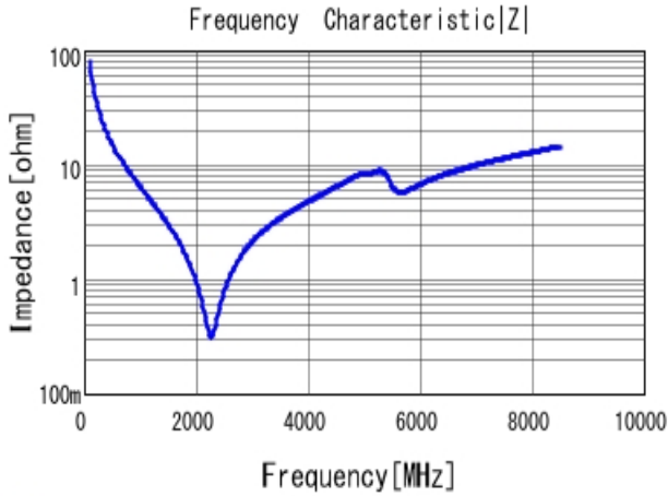
■ GRM0332C1H200JA01 |Z| DC0V, 20degC
