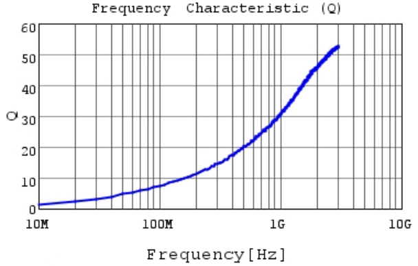
LQG15HZ1N2C02 Q
