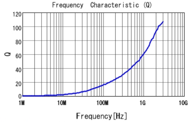
LQW15AN1N6D80 Q
