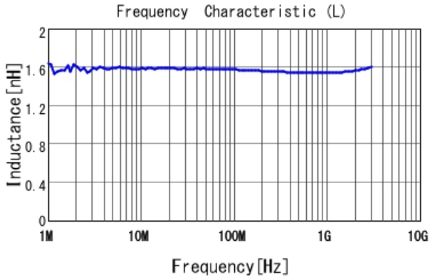
LQW15AN1N6D80 L
