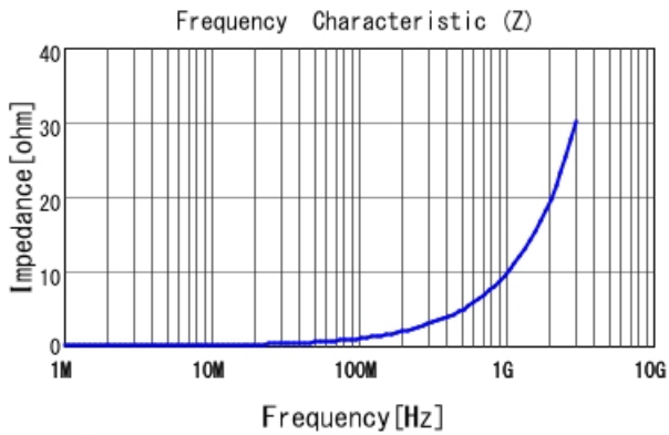
LQW15AN1N6D80 |Z|
