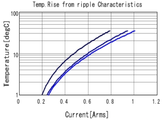
GRM1552C1H9R0DA01 Temp. rise ■ 700MHz ■ 1GHz ■ 2GHz
