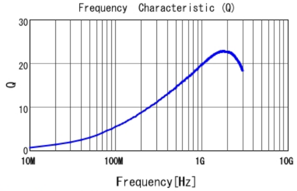
LQP03TG10NJ02 Q
