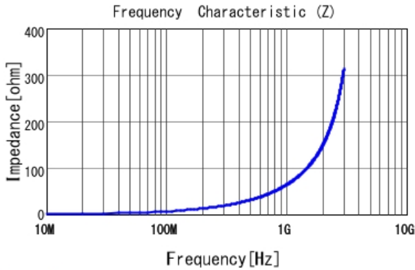
LQP03TG10NJ02 |Z|
