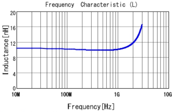
LQP03TG10NJ02 L
