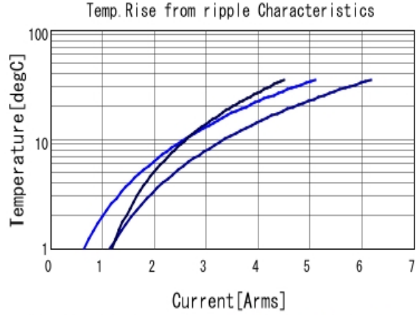
GRJ32ER71C226KE11 Temp. rise ■ 80kHz ■ 400kHz ■ 800kHz
