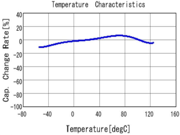
■ GRJ32ER71C226KE11 C-Temp. capchange, DCO. 0V, ACO. 5Vrm
