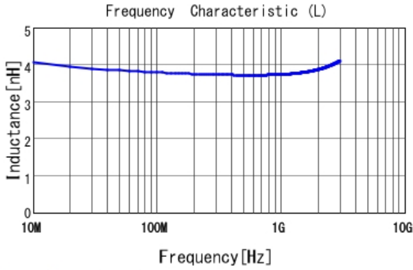
LQW15AN3N8C10 L
