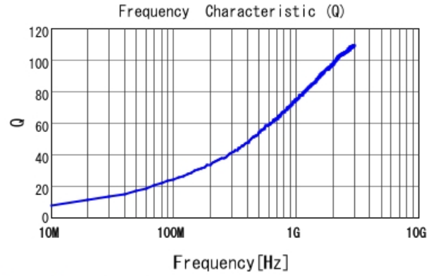
LQW15AN3N8C10 Q
