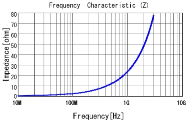
LQW15AN3N8C10 |Z|
