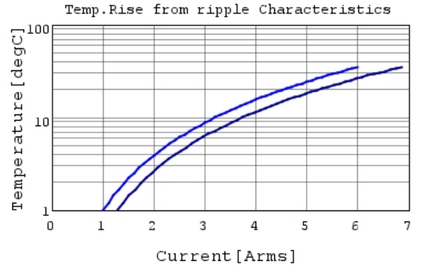
GCM32EC71H106KA03 Temp.rise — 80kHz
