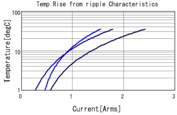
GRM31MR72A224KA01 Temp. rise — 300kHz — 600
