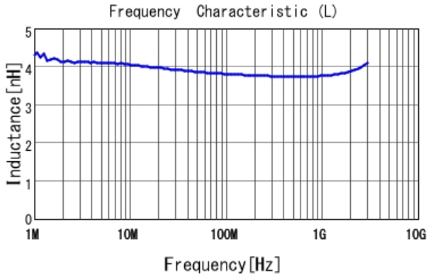
LQW15AN3N8G80 L
