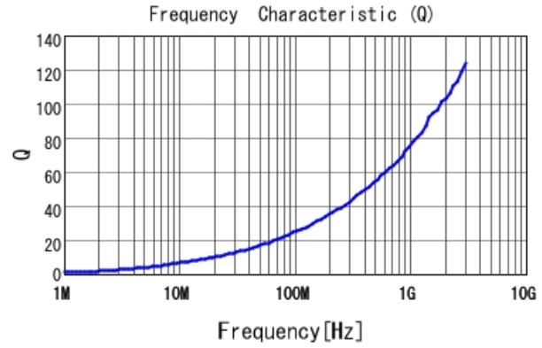
LQW15AN3N8G80 Q
