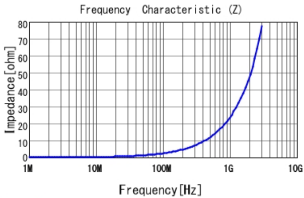
LQW15AN3N8G80 |Z|
