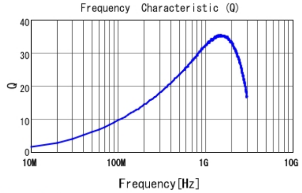
LQP03HQ22NH02 Q
