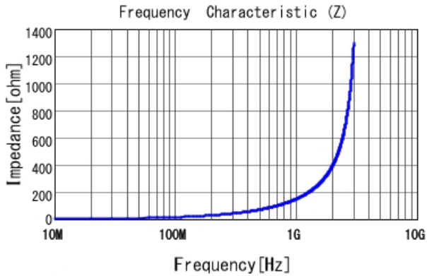
LQP03HQ22NH02 |Z|
