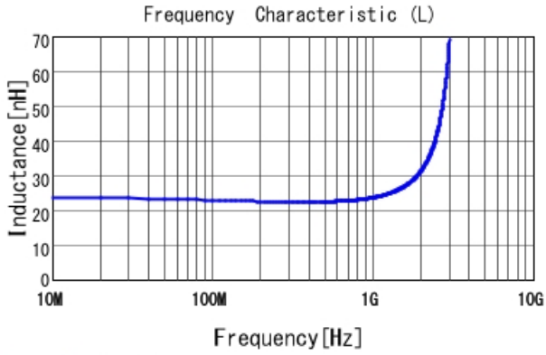
LQP03HQ22NH02 L
