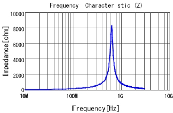
LQP03TNR24H02 |Z|
