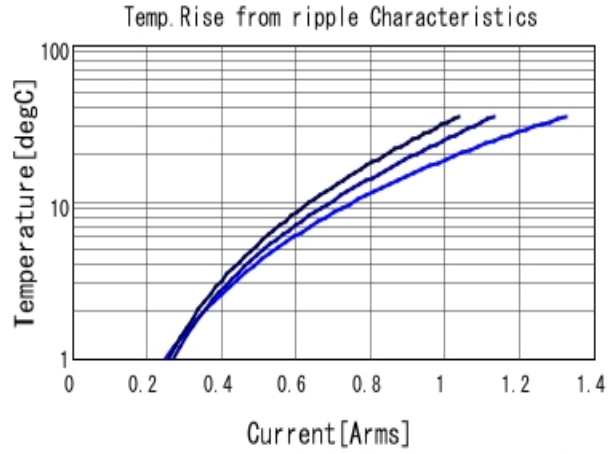
GRM1555C1H680JA01 Temp. rise ■ 200MHz ■ 500MHz ■ 700M
