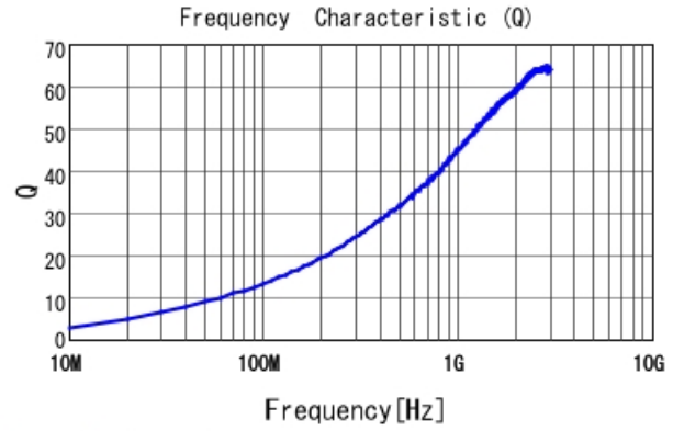
LQP03HQ4N3H02 Q
