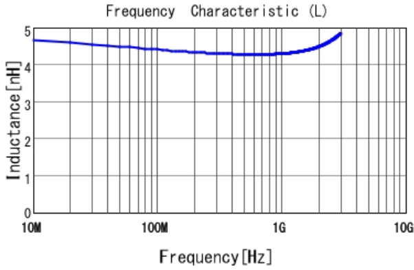
LQP03HQ4N3H02 L
