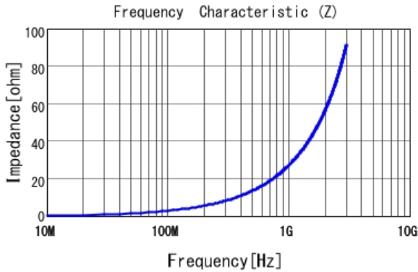
LQP03HQ4N3H02 |Z|
