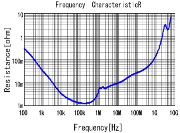
■ GRM32ER60J107ME20 R DCOV, 25degC
