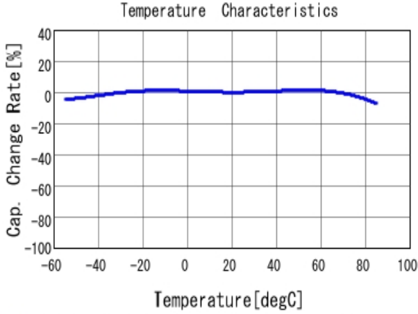
■ GRM32ER60J107ME20 C-Temp. capchange, DCO. 0V, ACO. 5Vrm
