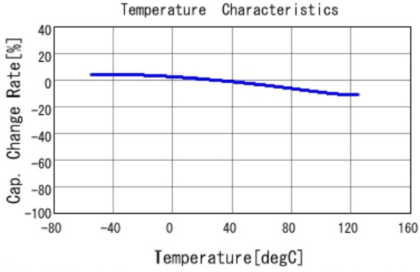
■ GRM033R71E682KE14 C-Temp. capchange, DCO. 0V, AC1. 0Vrm
